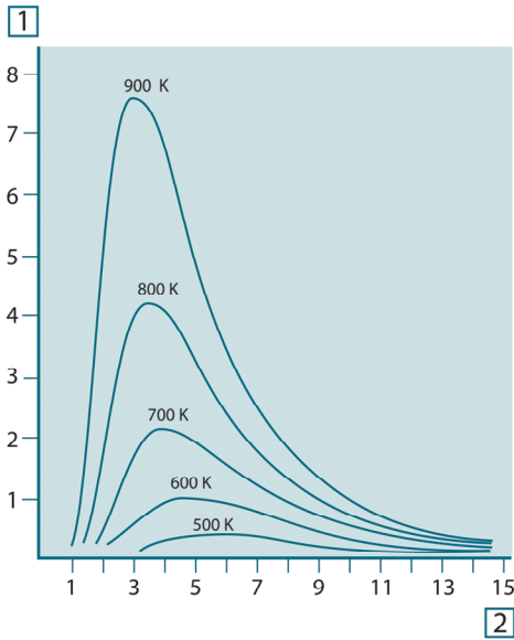
図 18.4 Planck の法則に従ってさまざまな絶対温度に対して描画された黒体スペクトル放射発散度。1 : スペクトル放射発散度 (W/cm 2 × 10 3 (μm))、2 : 波長 (μm)
