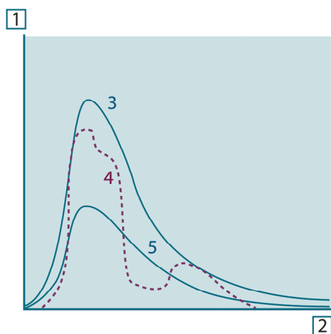
図 18.8 3 種類の放射体の分光放射率。1：分光放射率、2：波長、3：黒体、4：選択放射体、5：灰色体。
