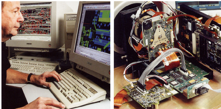
図 14.3 左: システムエレクトロニクスの開発。右: FPA 検出素子のテスト
