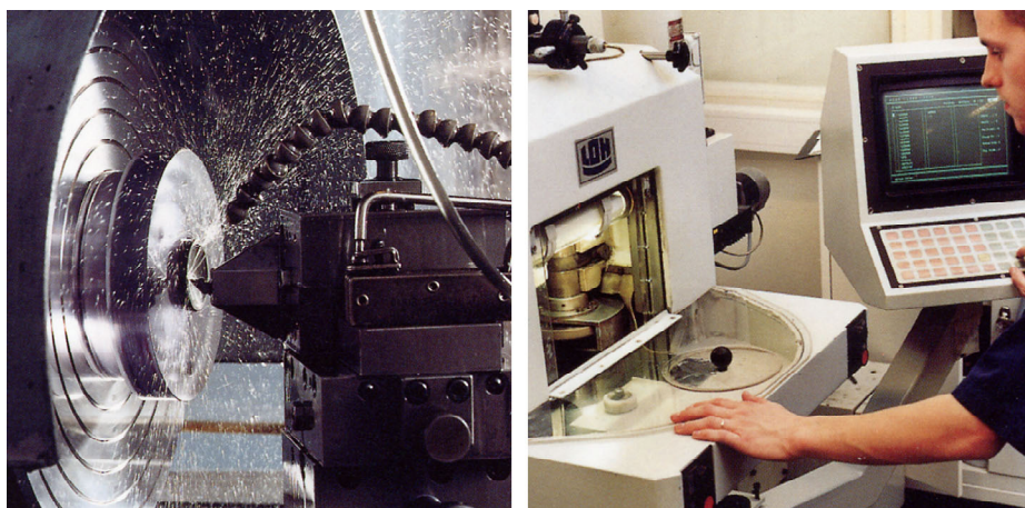
図 14.4 左: ダイヤモンド旋盤。右: レンズ磨き
