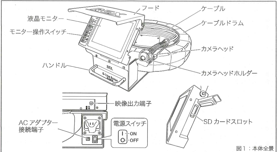
図1: 本体全景
