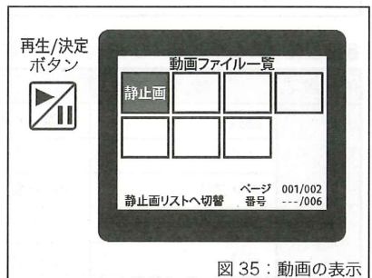
図 35：動画の表示
