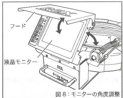
図8：モニターの角度調整
