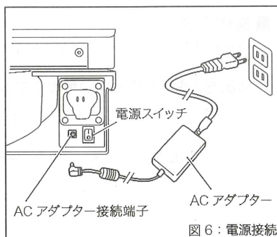
図6：電源接続
