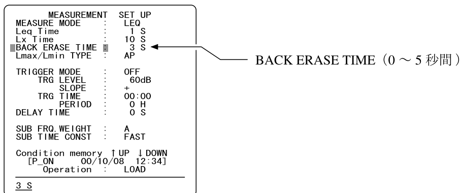
メニュー SET UP 画面
