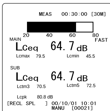
リコール画面
