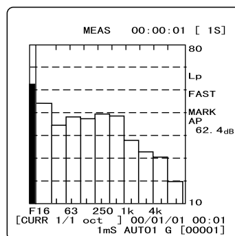
1/1 オクターブ分析画面
