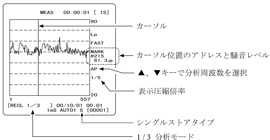
レベル対時間リコール画面
