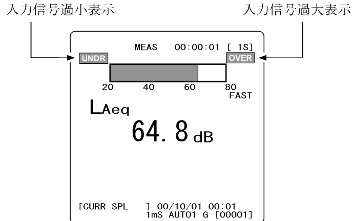
騒音レベル測定画面
